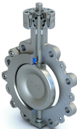
4-Cx Anflanschgehäuse
