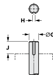
Axe avec Rainure de Clavette ≥ DN 350
